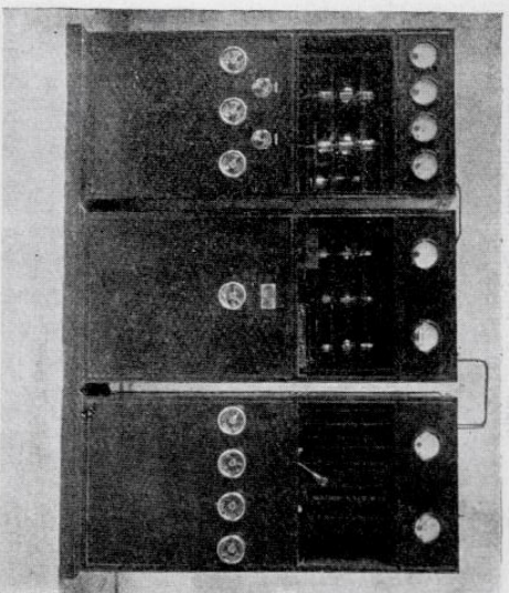
První československá rozhlasová stanice ve Starých Strašnicích. Première station de radiodiffusion de Praha (Strašnice) installée en 1925.
